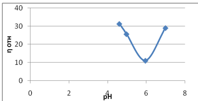
Рис. 2. Зависимость относительной вязкости 10%-ного раствора ПАК от pH
