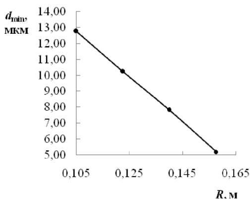
Рис. 3. Распределение минимального размера улавливаемых частиц по сечению первой ступени при \rho_{ч} = 2100 кг/м 3
