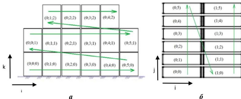
Рис. 2. Иллюстрация стратегий заполнения контейнерной площадки:
