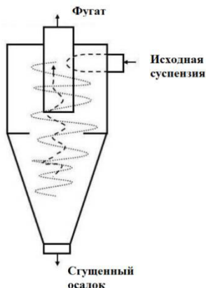
Рис. 1. Схема гидроциклона
