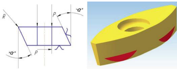
Рис. 2. Конструкция сменной режущей пластины
