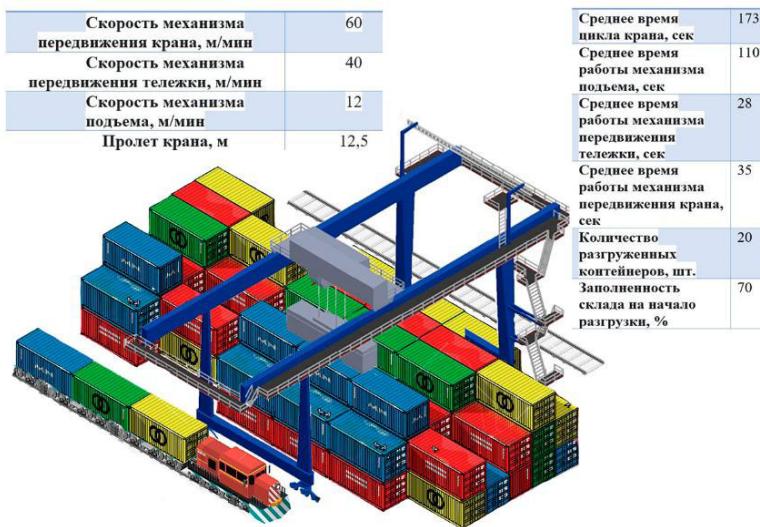
Рис. 2. Расчет имитационной модели крана
