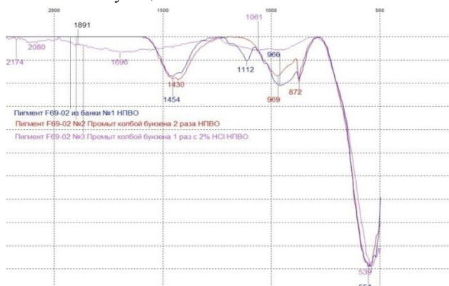
Рис. 2. ИК-спектр пигмента без промывки, промытого дистиллированной водой, а также 2%-ным соляным раствором
