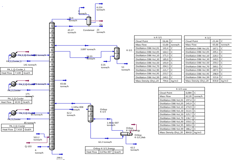
Рис. 1. Модернизированная модель стрипинг-секции К-3/3 установки ЭЛЮУ-АТ-4 в расчетной программе Petro-SIM
