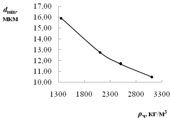
Рис. 2. График зависимости минимального размера улавливаемых частиц от плотности частиц дисперсной фазы при R = R_0
