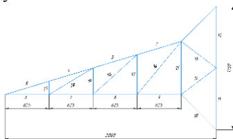
Рис. 1. Раскосная ферма
